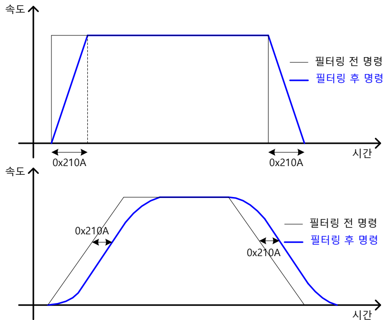
위치 명령 평균 필터 시정수(0x210A)를 이용한 위치 명령 필터
