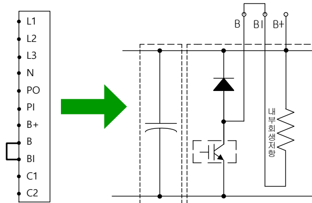
내부 회생 저항 사용 시 배선 방법
