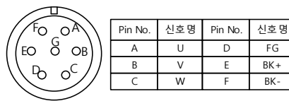
Plug : MS3102A24-10P
