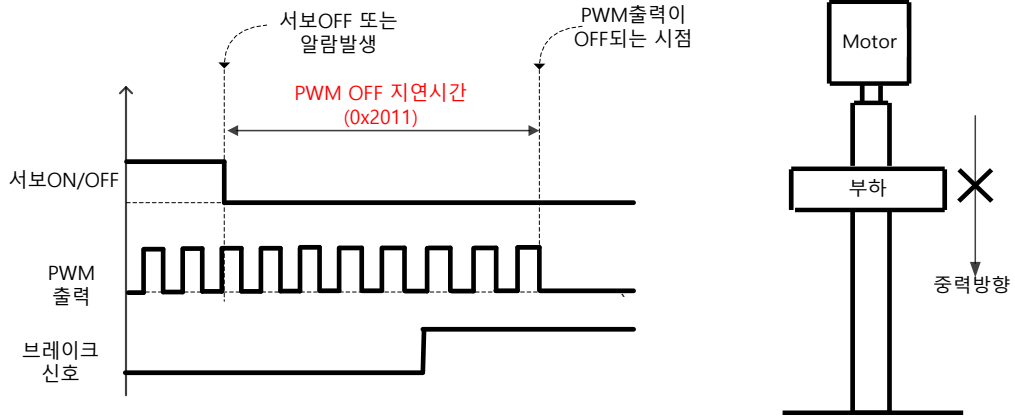
(1) 브레이크 신호가 먼저 출력되고 PWM 출력이 OFF 되는 경우
