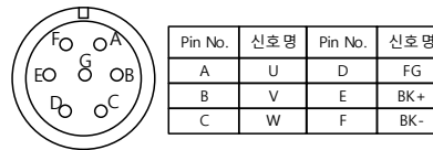
Plug : MS3102A20-15P
