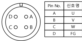
Plug : MS3102A22-22P
