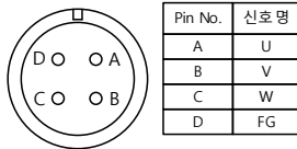
Plug : MS3102A20-4P
