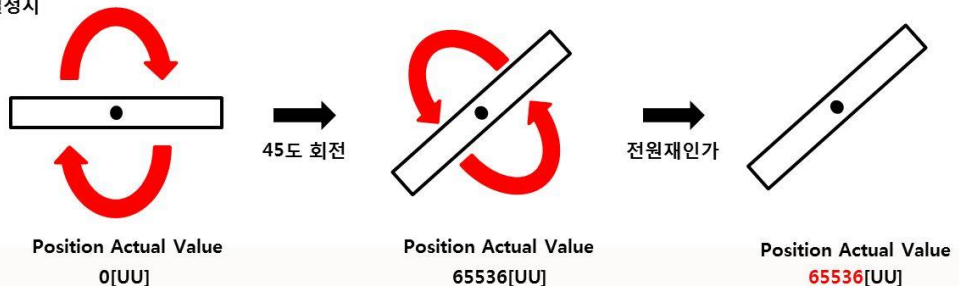
절대치 싱글턴 엔코더 0 설정시
