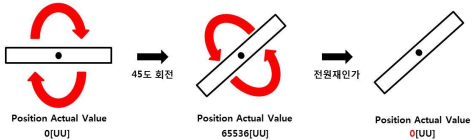
절대치 싱글턴 엔코더 1 설정시
